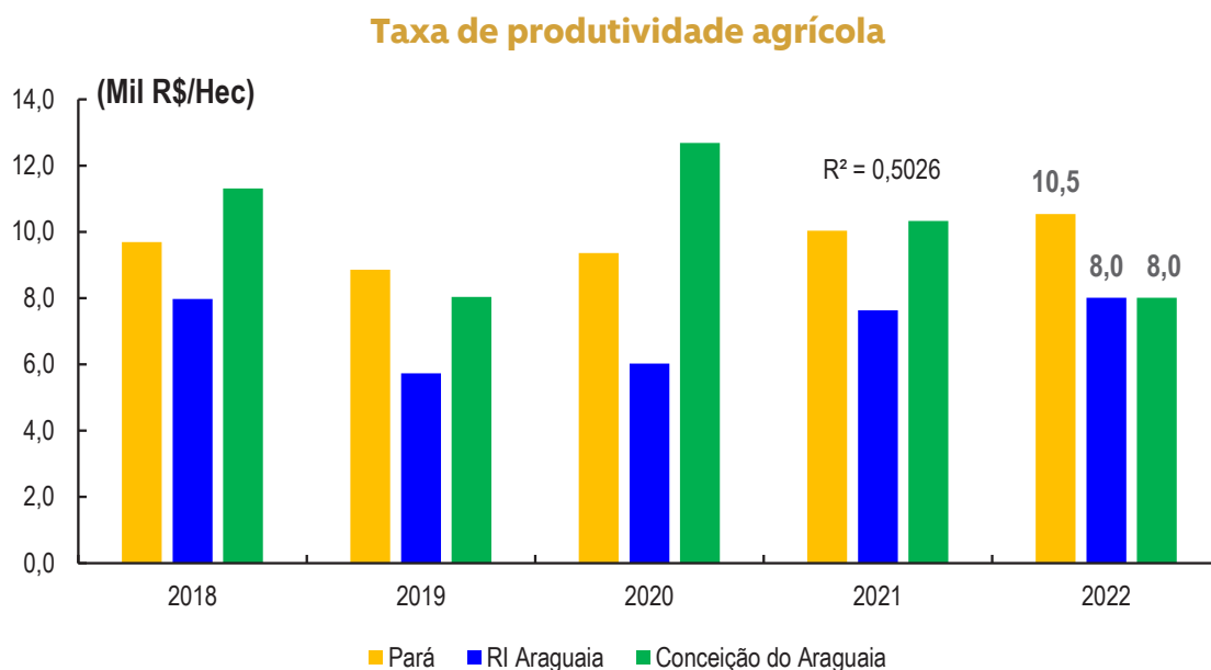
Gráfico 04: Taxa de produtividade agrícola, Pará, Região de Integração Araguaia e Conceição do Araguaia, 2018 a 2022.
